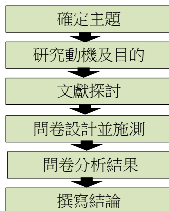
圖 1 研究架構圖
